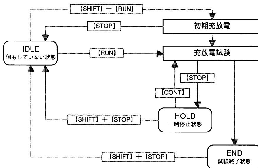
図2-2 CYCLE運転
