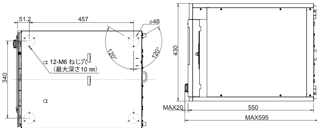
A矢視キャストねじ位置図
