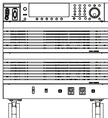
A矢視キャストねじ位置図
