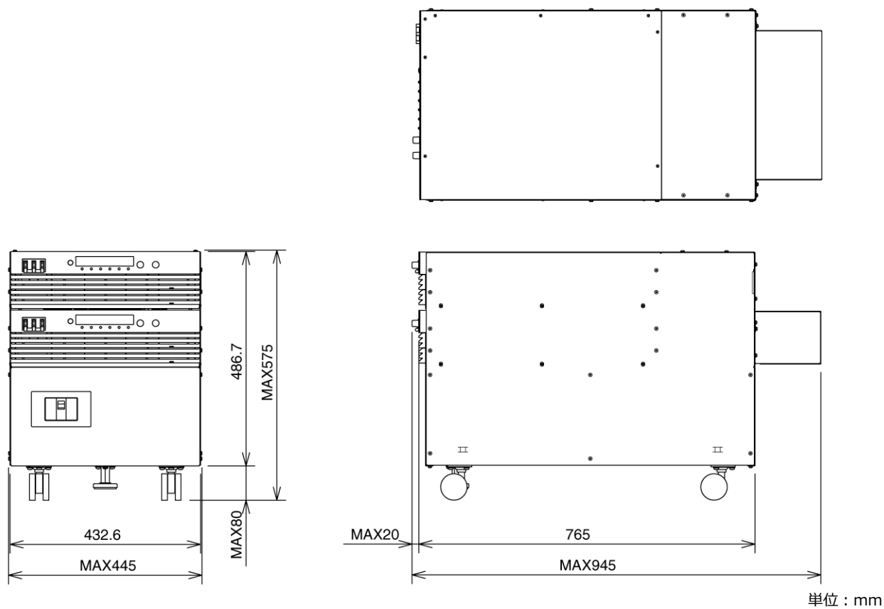
PAT-TMXシリーズ 16 kWシステム 外形寸法図
