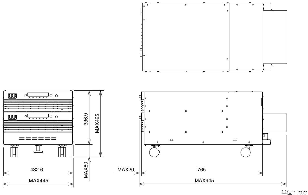
PAT-TMシリーズ 16 kWシステム 外形寸法図
