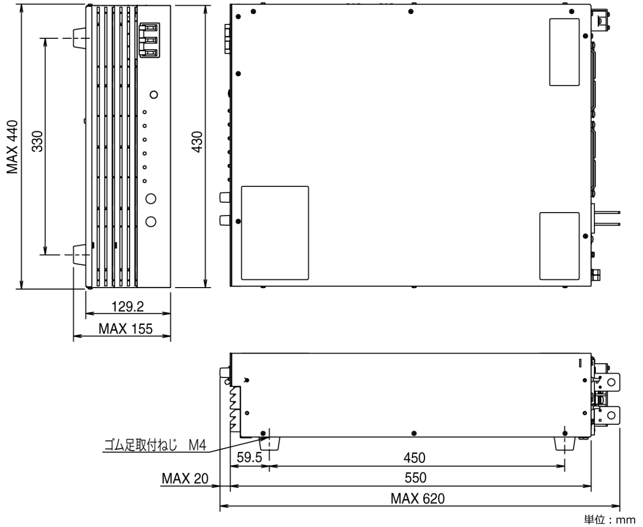
PAT-Tシリーズ 外形寸法図
