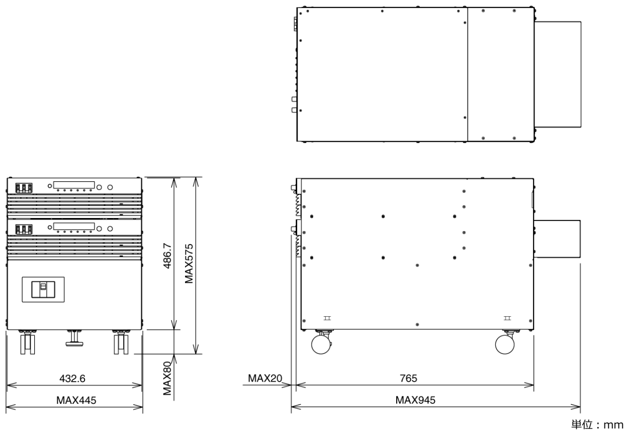
PAT-TMXシリーズ 16 kWシステム 外形寸法図
