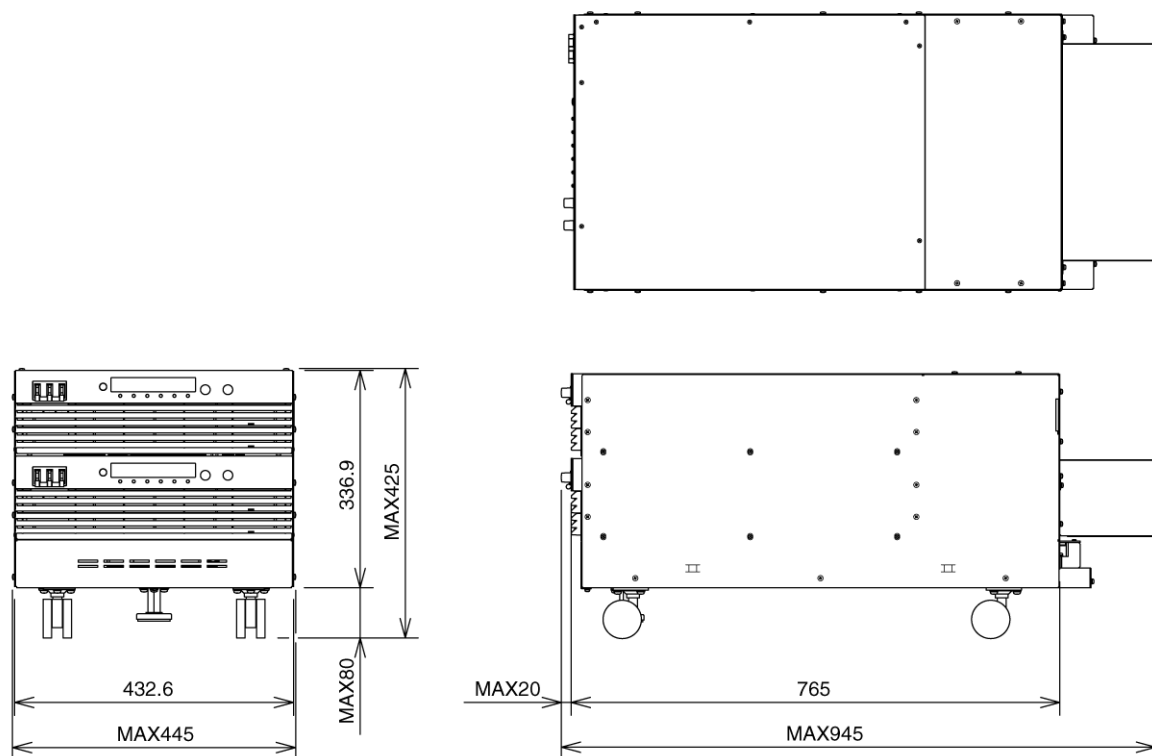
PAT-TMシリーズ 16 kWシステム 外形寸法図
