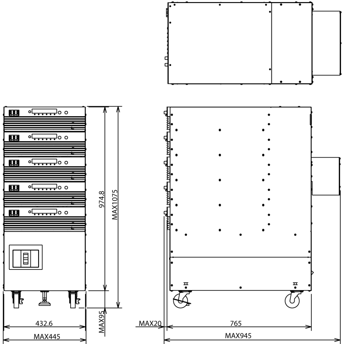
PAT-TMXシリーズ 40 kWシステム 外形寸法図
