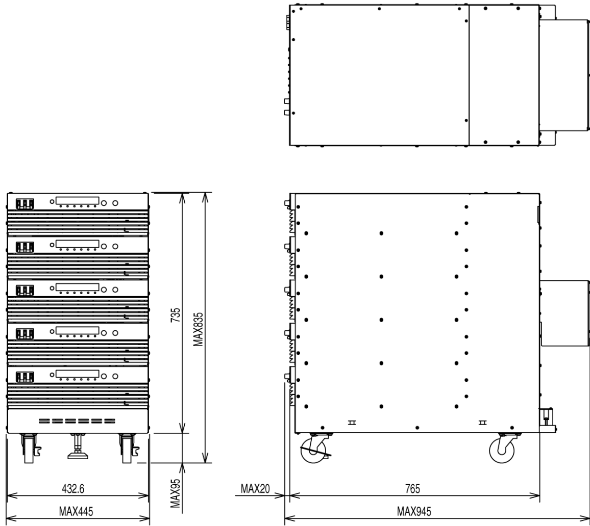
PAT-TMシリーズ 40 kWシステム 外形寸法図
