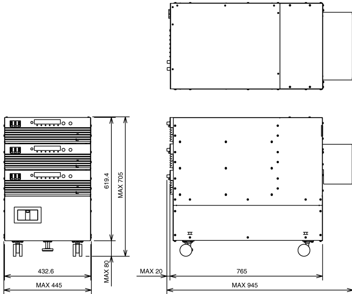
PAT-TMXシリーズ 24 kWシステム 外形寸法図
