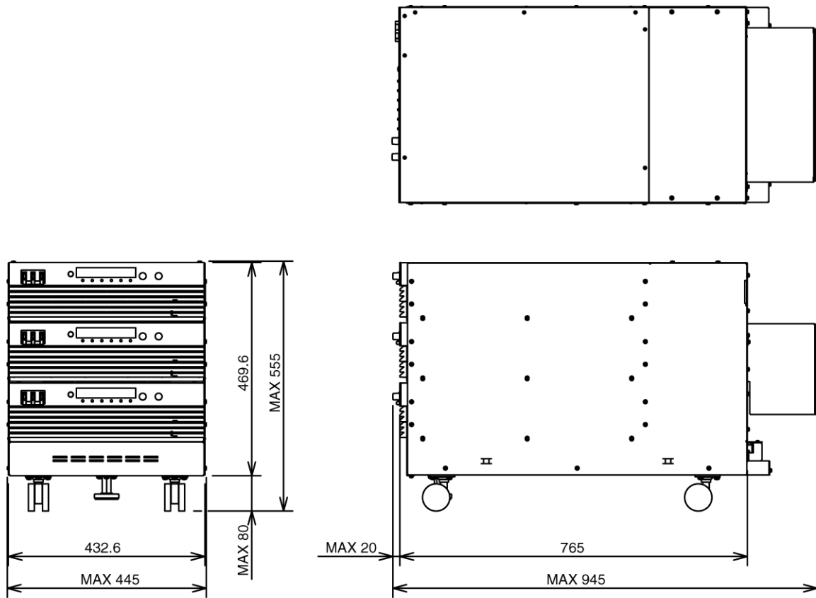
PAT-TMシリーズ 24 kWシステム 外形寸法図
