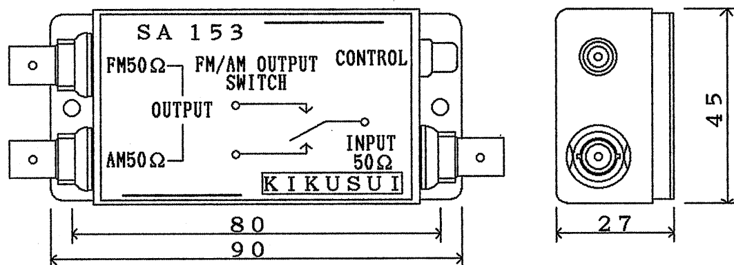
第 9-14 図 外形図
